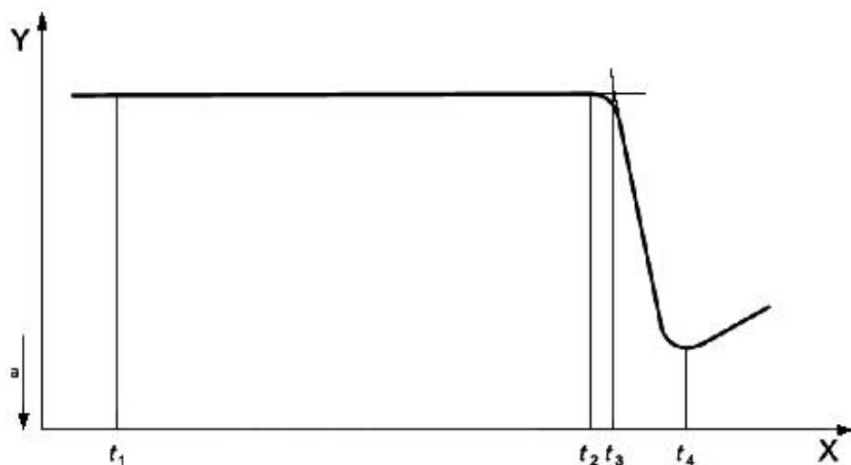
Рисунок 4 - Типичная кривая ДСК при определении термостабильности
