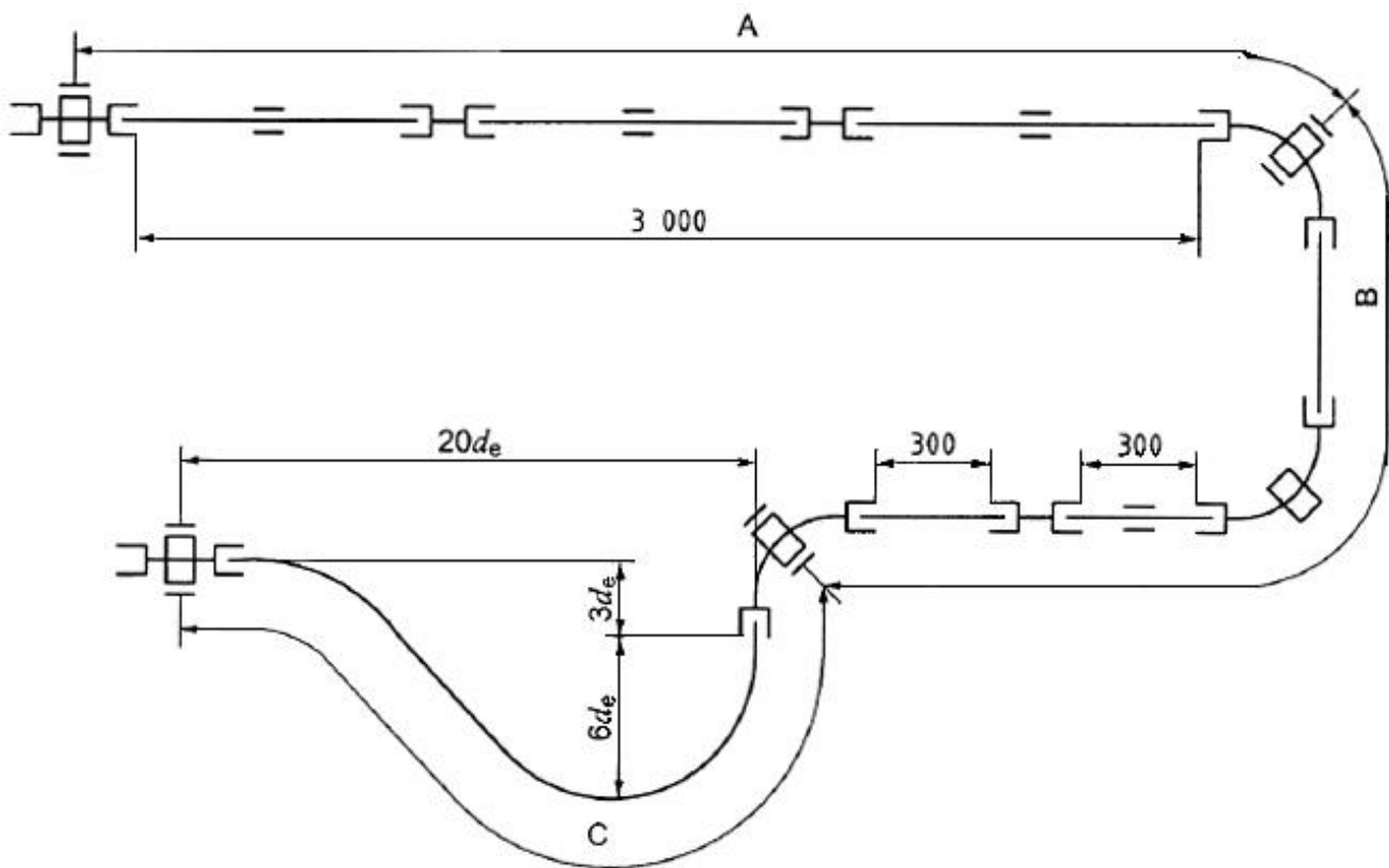
Рисунок 5 - Схема испытательной сборки для проверки стойкости соединений при переменной температуре
