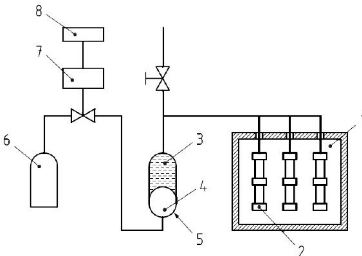
Рисунок 6 - Схема стенда для проверки стойкости соединений при переменном давлении
