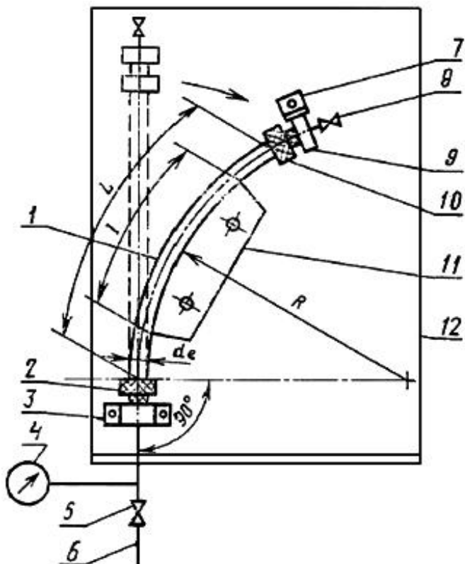
Рисунок 7 - Схема проверки герметичности соединений при изгибе и действии внутреннего давления
